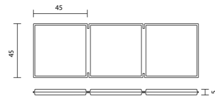
Sitz / Rückenissen back rest / seat cushion cousin d'assise / dossier ■ 210 100 TU8013 ■ 210 100 D10235 ■ 210 100 TU3669 ■ 210 100 D10160 ■ 210 100 TU8001 ■ 210 100 DSJ352 ■ 210 100 TU3667 ■ 210 100 DSJ355
